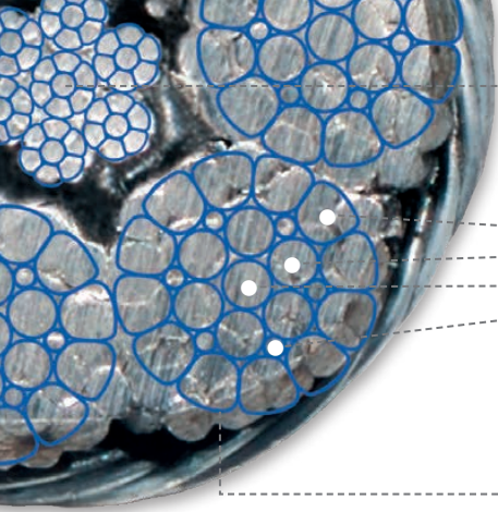
6 gevlochten buitendraden met elk 25 draden
