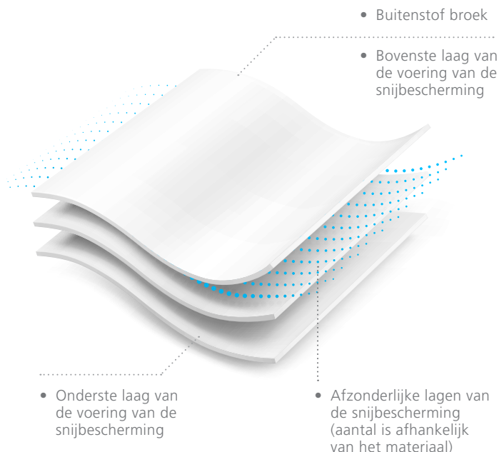
Opbouw van de snijbeschermingslagen
