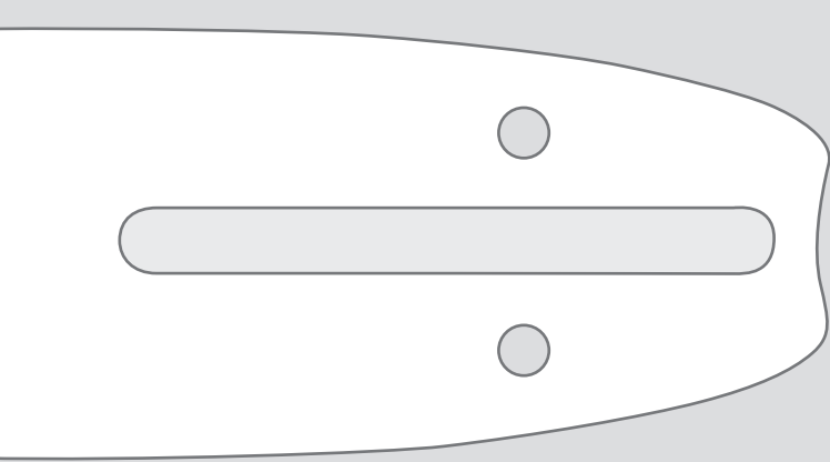
AANSLUITING: A041, Z041 Dolmar, Makita, Echo en anderen 3/8" hobby 1,1 mm met 1,3 mm
